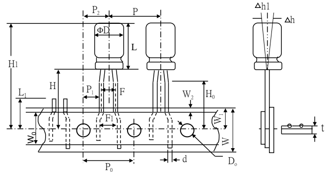
Fig.4( \Phi 10 )
