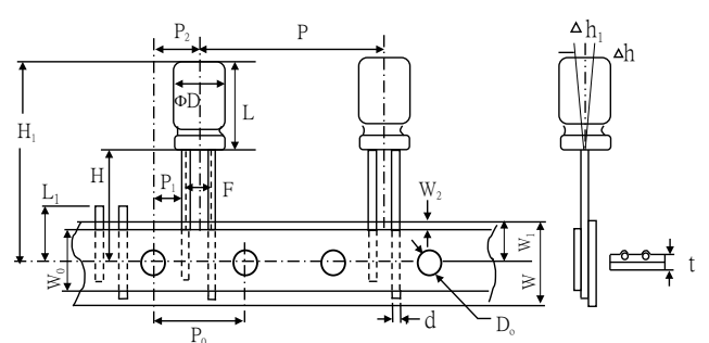
Fig.6( \Phi 16 )
