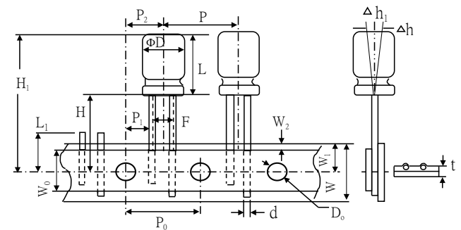
Fig.6( \Phi 16 )
