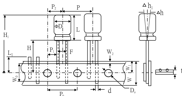
Fig.5( \Phi 12-13 )
