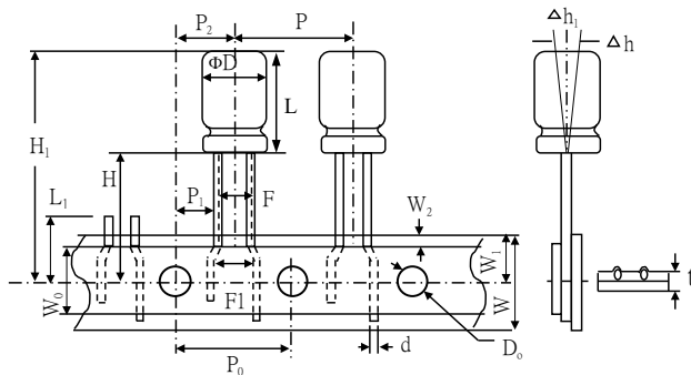
Fig.5( \Phi 12-13 )
