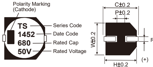
Fig.2 \varnothing D \geq 12.5\text{mm}
